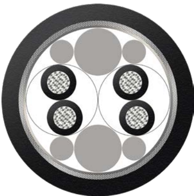
BizLink SeaLine® BWTS Kabel 2x2x0.75 VZN BK Bestell-Nr.: L45551-D22-K16
