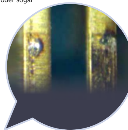
Kontaktabbrand in der Anschlussstechnik – hier eine RJ45-Buchse (aus IEC 62652)
